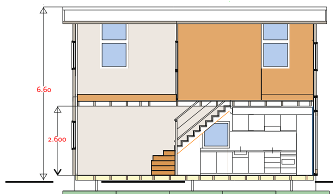
doorsnede A-A vanuit zuid
